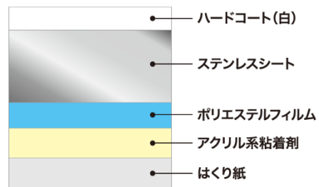
テープ構成
